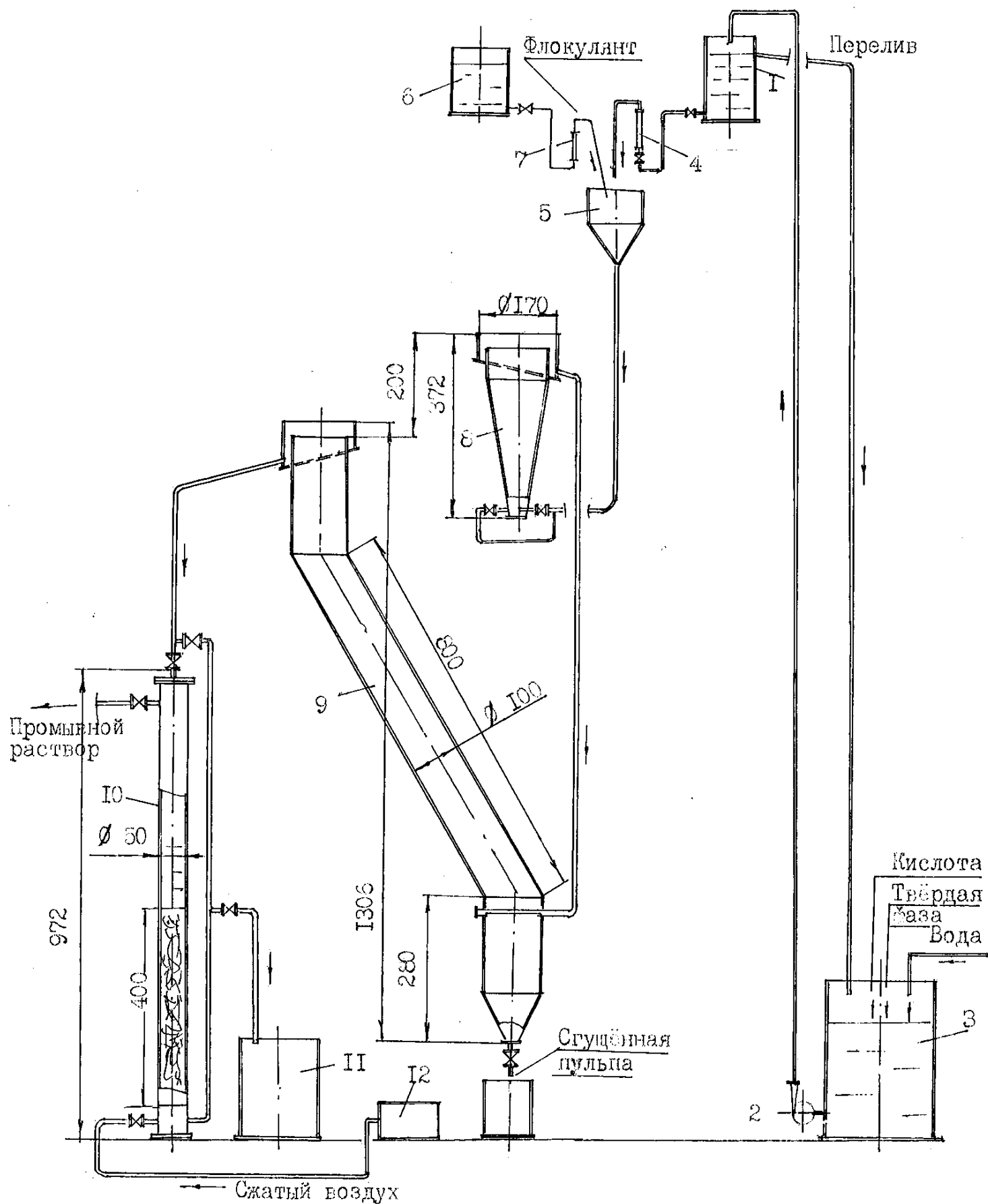
Схема полупромышленной установки для осветления растворов
