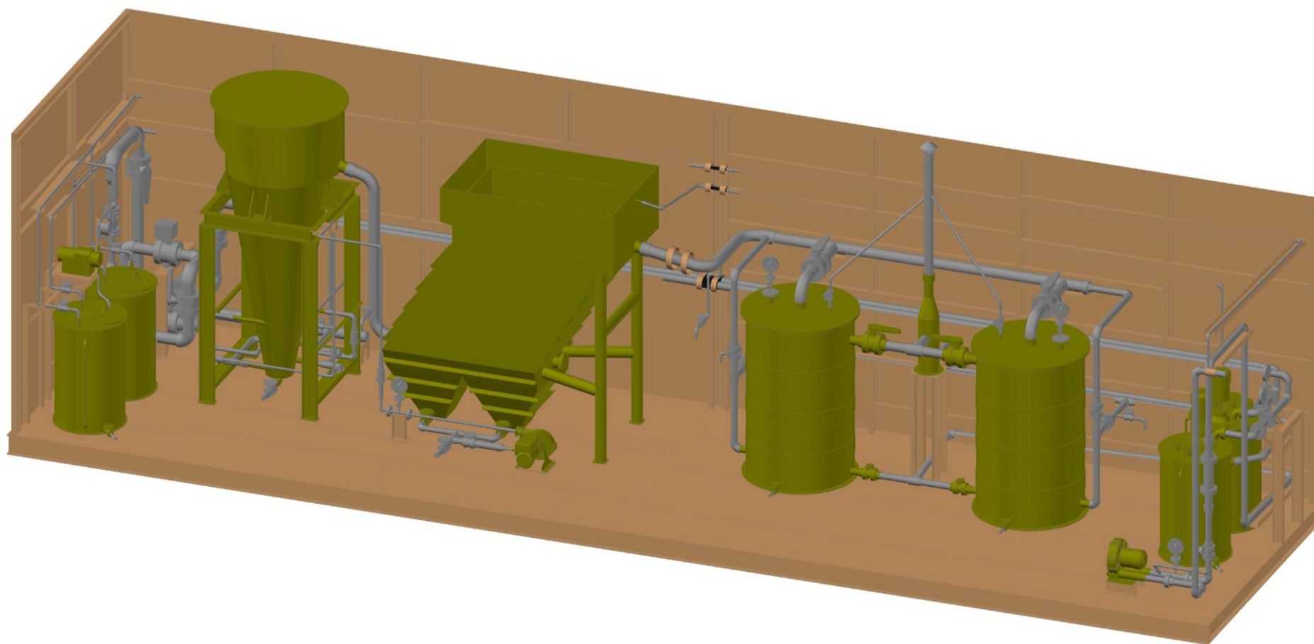
Монтажная схема установки для осветления растворов на этапе закисления блоков залежи
