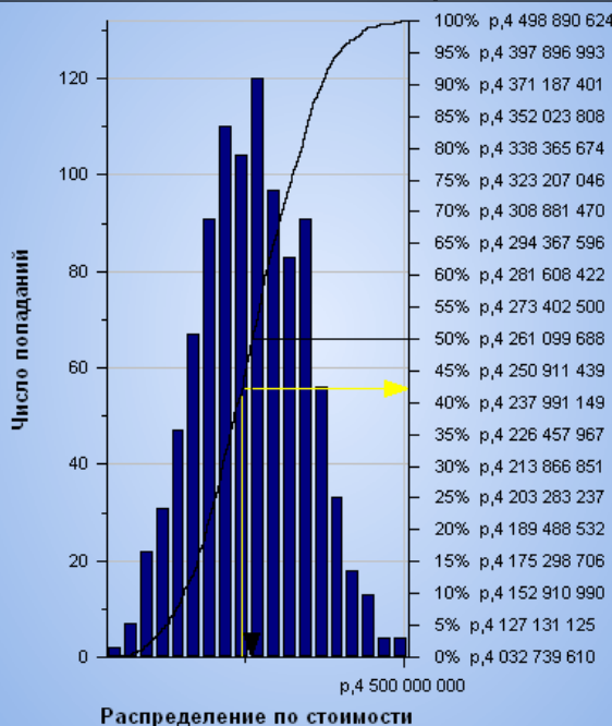
Гистограмма распределения стоимости проекта
